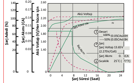
Voltaj ve Şarj Süresi
